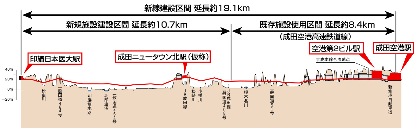
縦断面図
